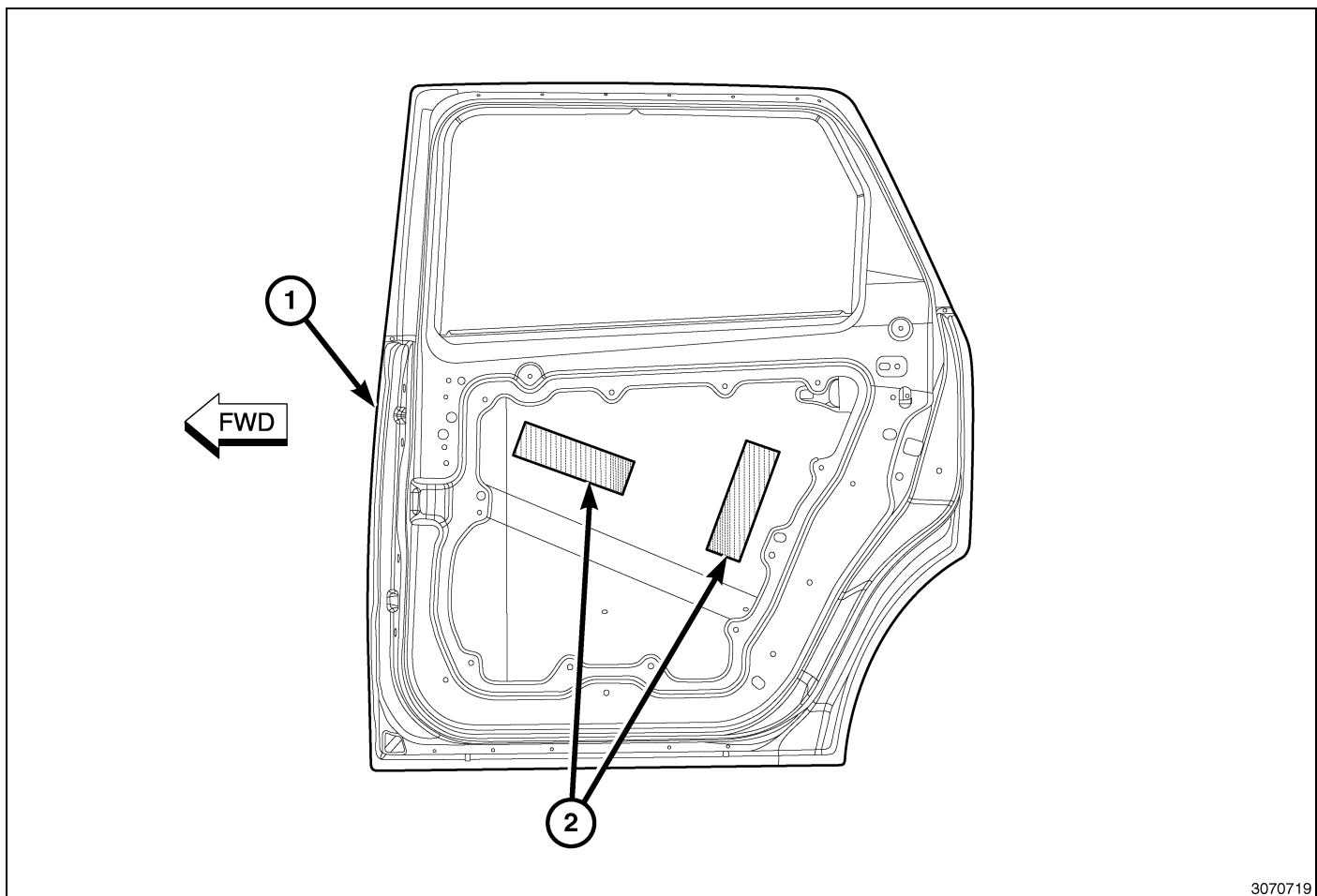
Fig. 27 Rear Door
