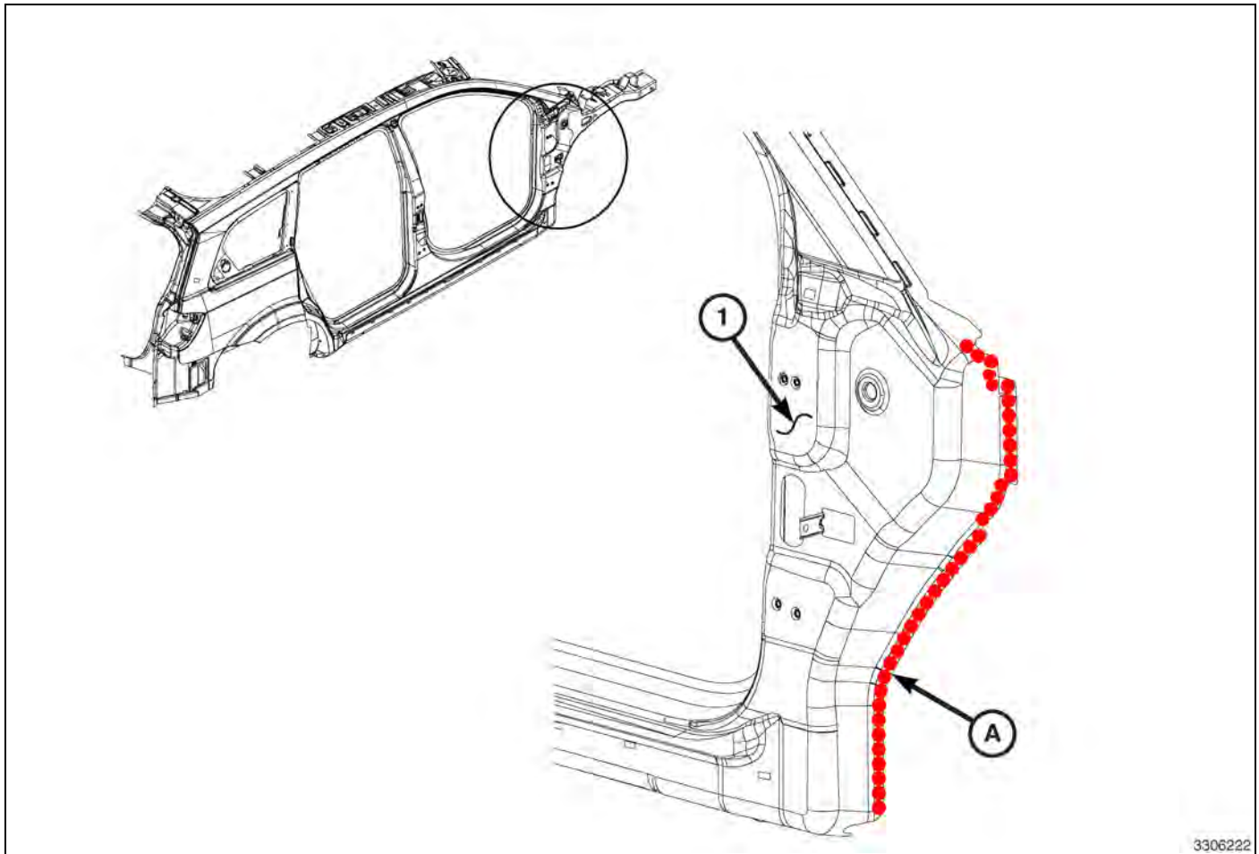
Fig. 61 Body Side Aperture A-pillar
