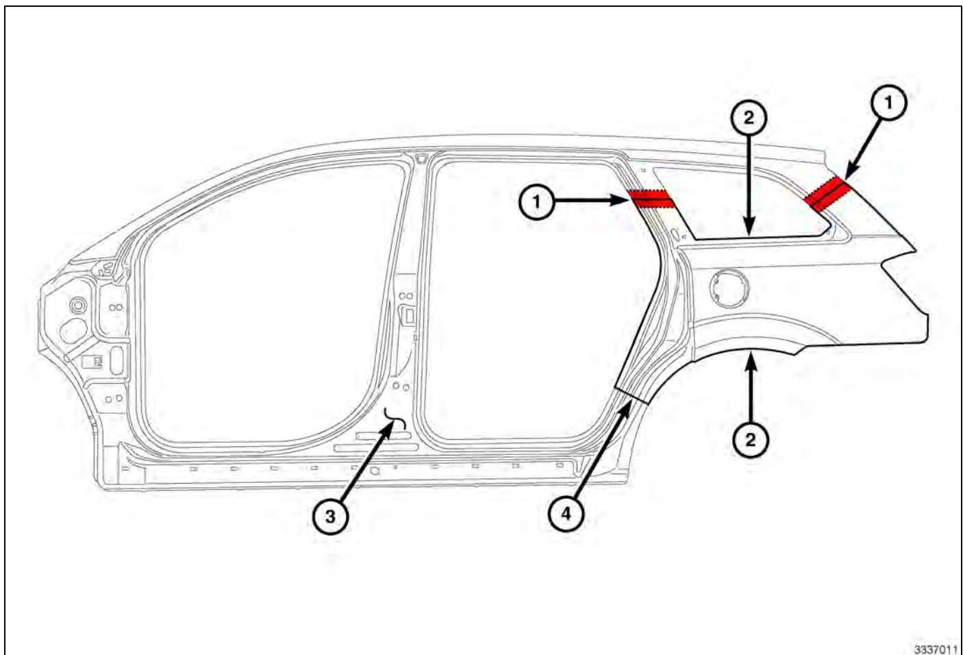
Fig. 11 Body Side Aperture
