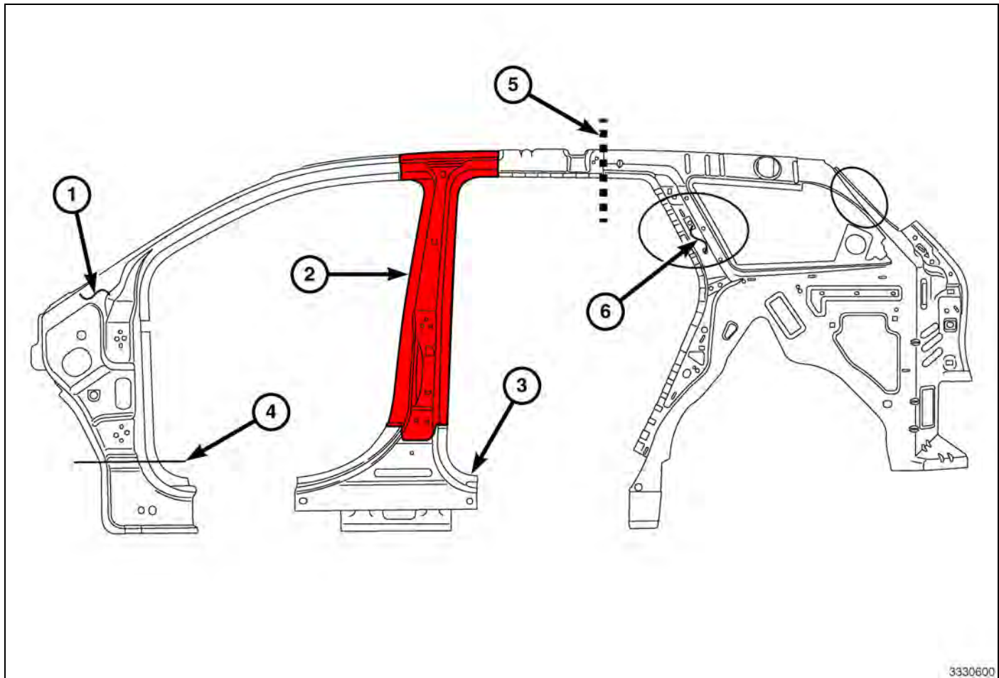
Fig. 22 Inner Body Side
