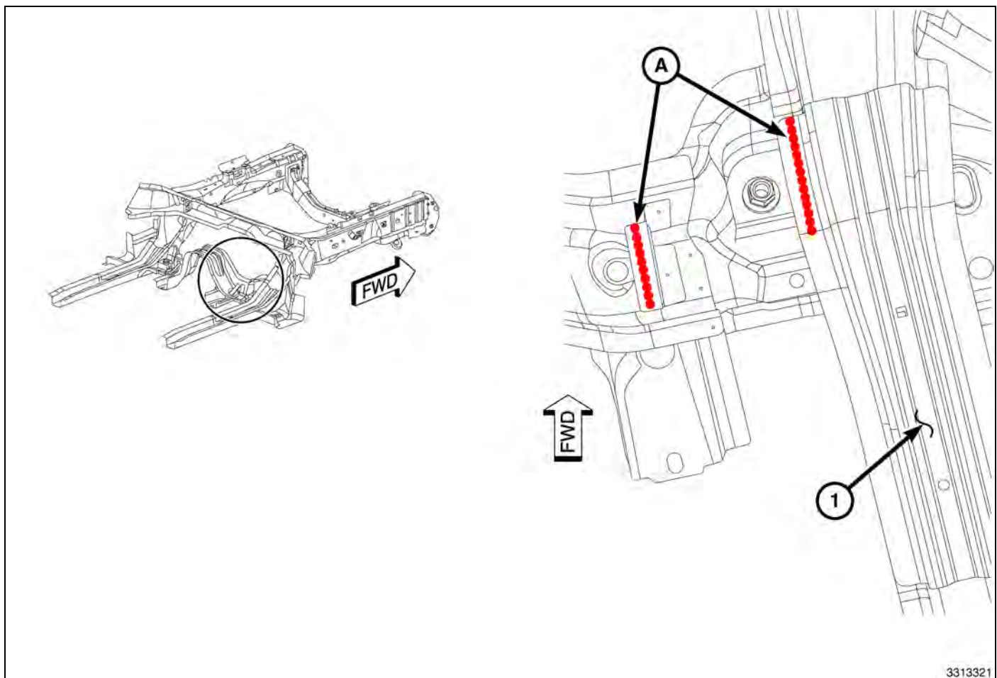
Fig. 66 Dash
