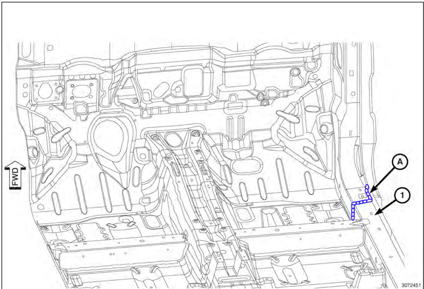
Fig. 35 Inner Sill
