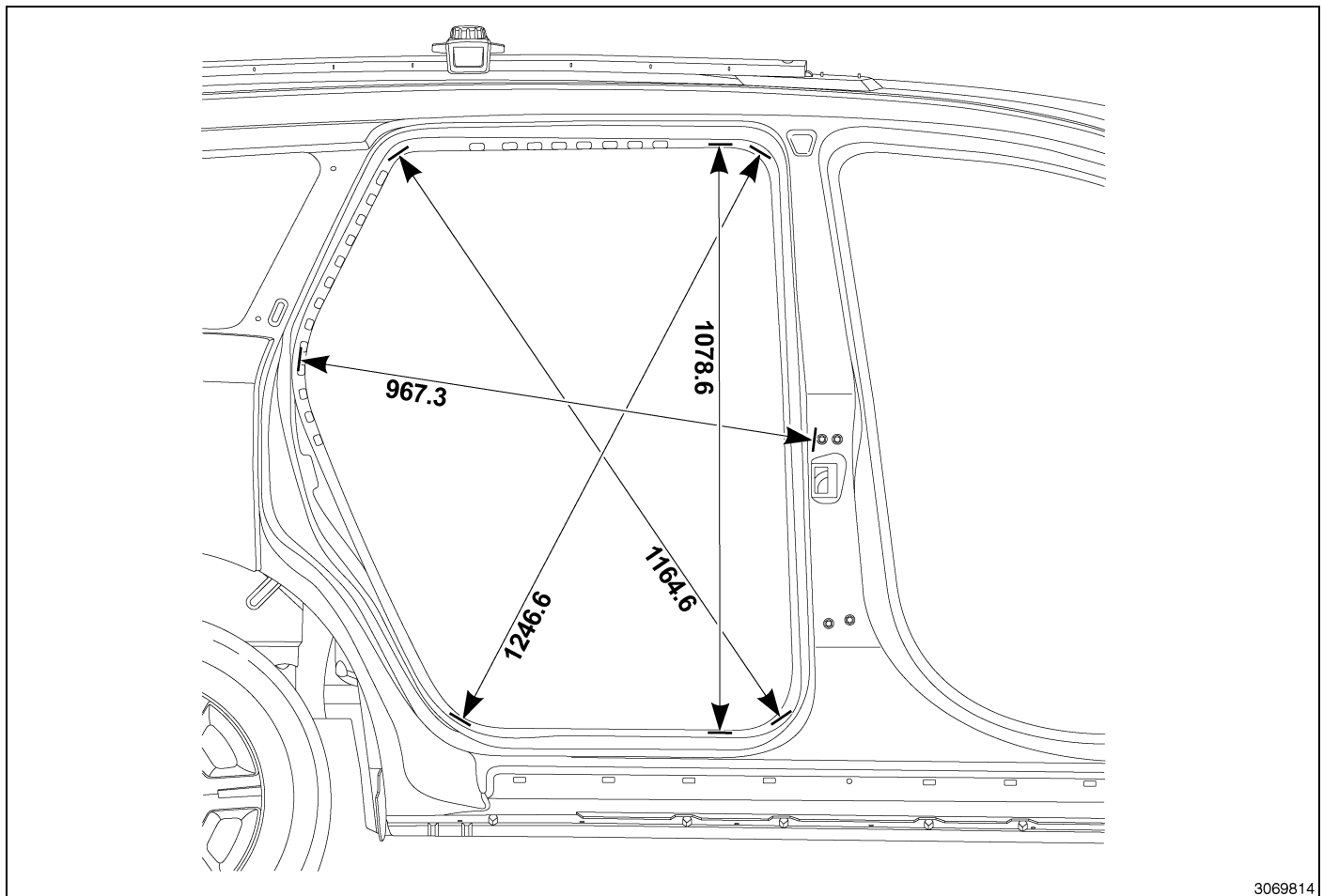
Fig. 3 Rear Door
