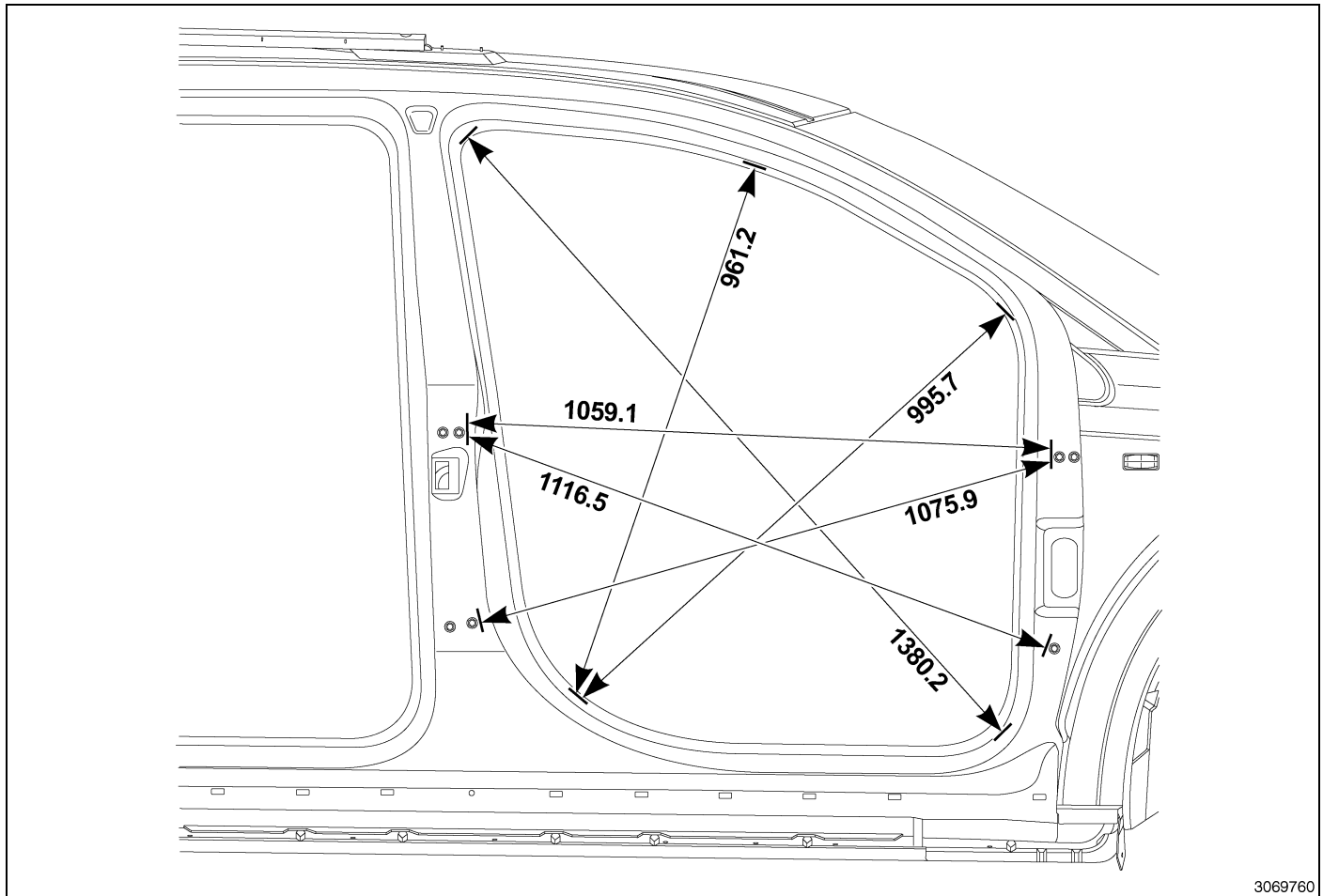
Fig. 2 Front Door
